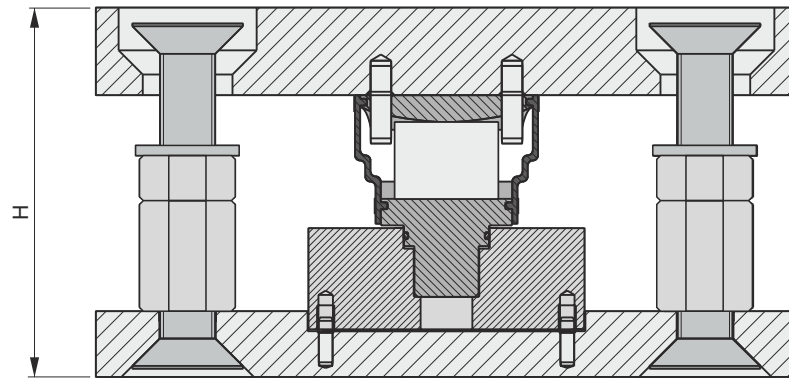
A - A
