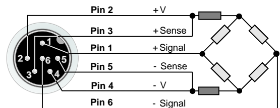
DMS-Anschluss in 6-Leiter-Technik
