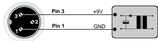
Spannungsversorgung 9V/8W
