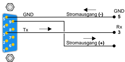
Druckerausgang oder Großanzeige über RS-232 oder 20mA Stromschleife
